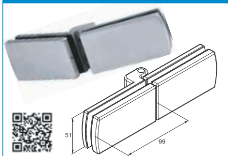
Apakšējais savienojuma fiksators 51-28.29.055-0
