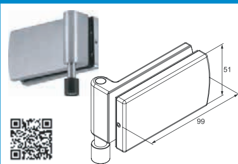
Augšējais savienojuma ritenis 51-28.29.054-0
