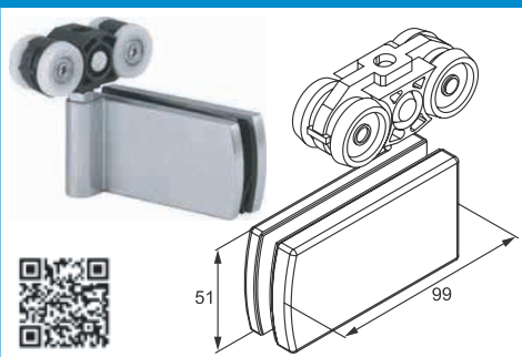
Apakšējais savienojums ar aizverēju 51-28.29.053-0
