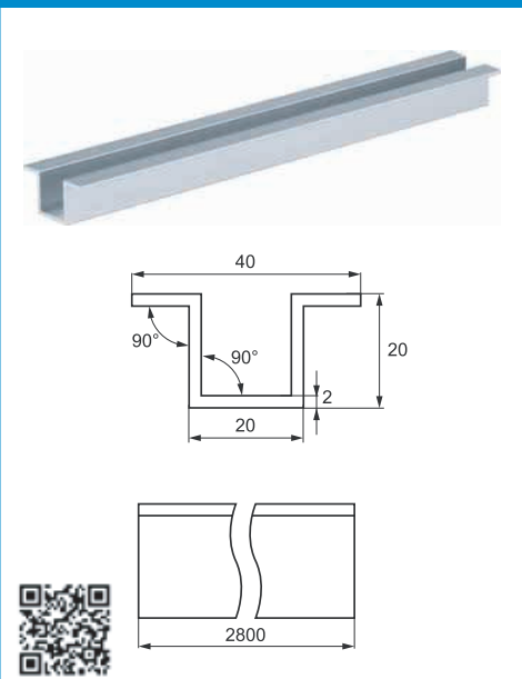
Apakšējā iefrēzējamā vadotne, L-2800 mm 16-28.25.221-1
