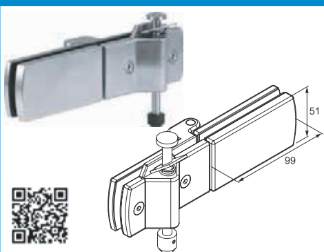
Apakšējais nobeigums 51-28.29.056-0
