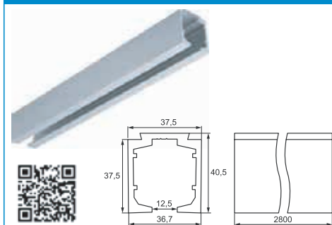
Augšējā vadula, L-2800 mm 16-28.25.220-1
