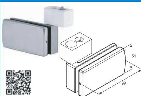
Augšējais nobeigums 51-28.29.057-0
