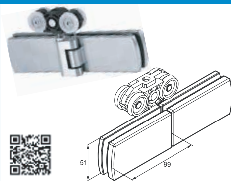
Augšējais nobeigums 51-28.29.057-0
