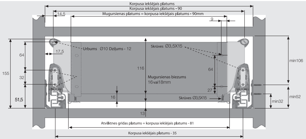
1. Atvilktnes grīda
