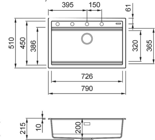
Tehniskais zīmējums
