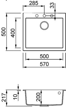
Tehniskais zīmējums
