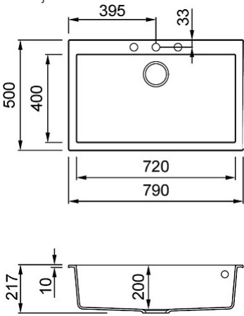
Tehniskais zīmējums
