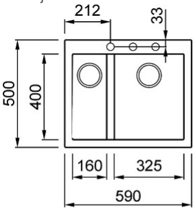
Tehniskais zīmējums
